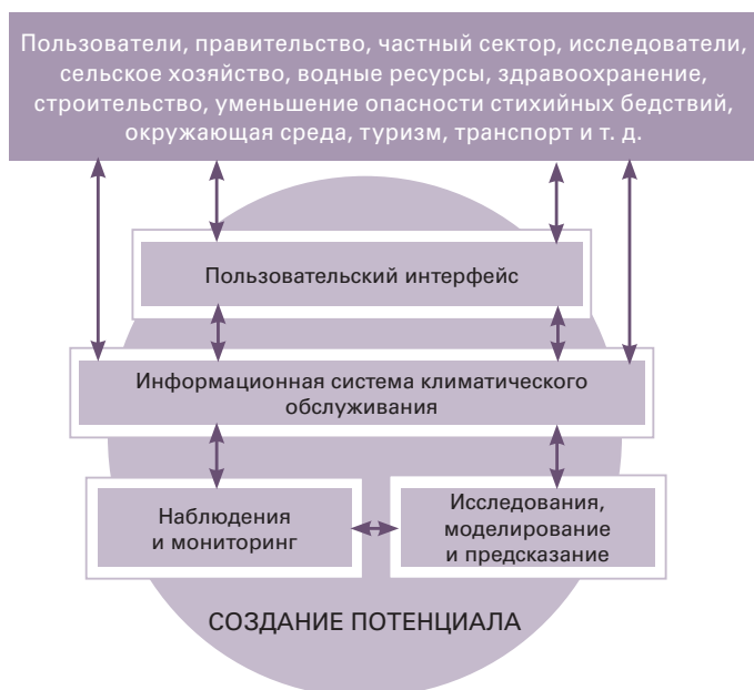
Схема компонентов Глобальной рамочной основы для климатического обслуживания с элементом создания потенциала в рамках всех других компонентов и между ними
